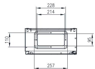
SECTION AY-AY
