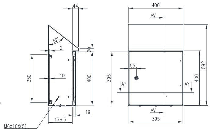
SECTION AV-AV
